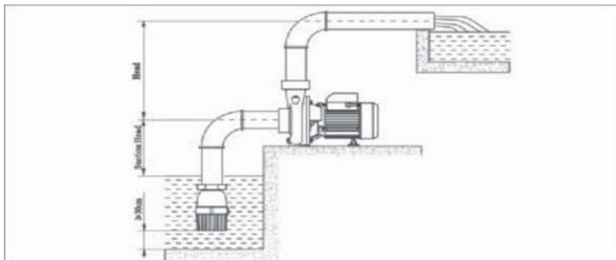
Schema instalarii
